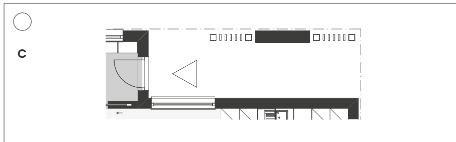
Versión con marquesina de entrada
