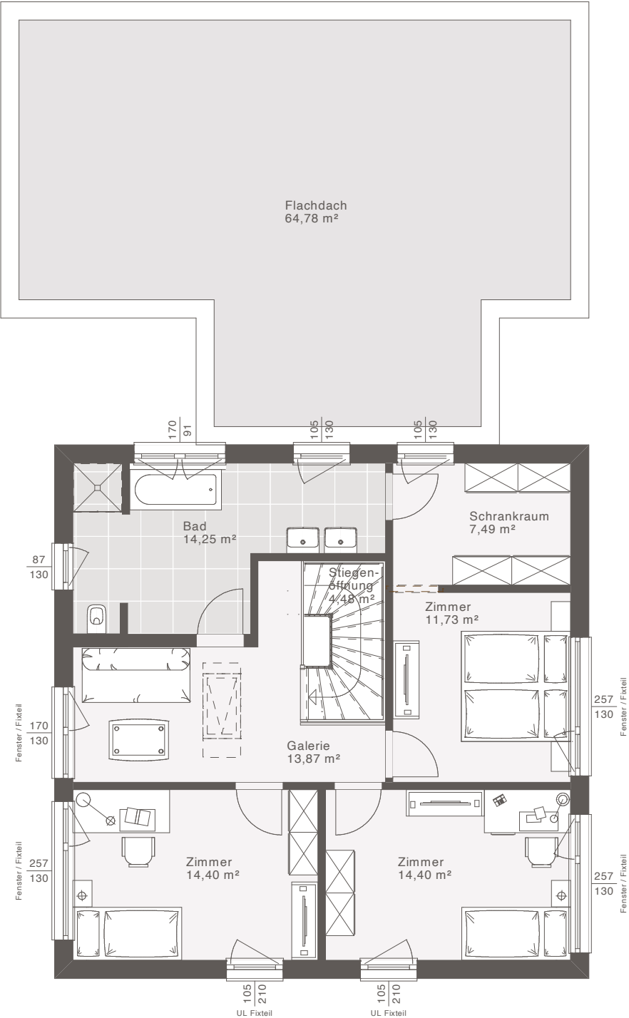
Planta alta Superficie útil interior: 80,62 m² Ejemplo de diseño | Cubierta plana
