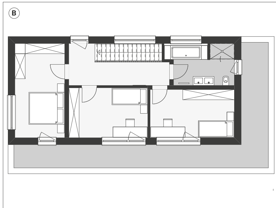
Versión con pérgola de terraza y marquesina de entrada
